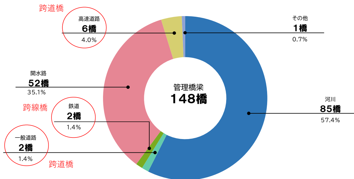
図 9 交差状況
